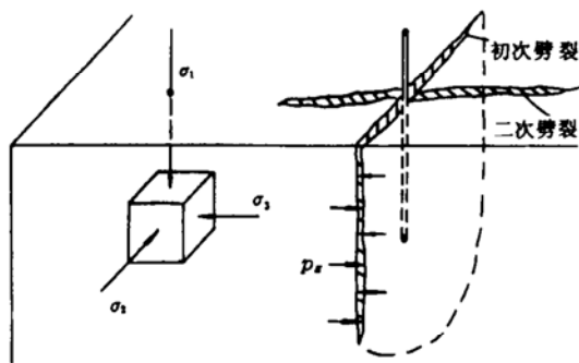
图2 土体中的应力和劈裂面
