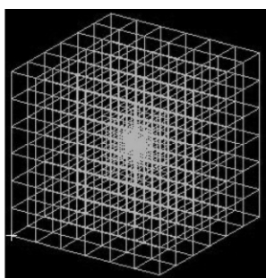
图1 爆源周围单元的划分方式
