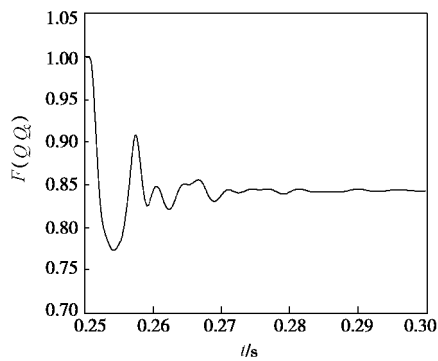
图6 爆源周围岩体破坏时内能变化图
