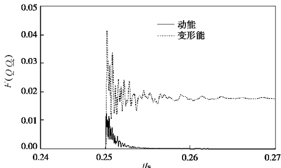
图 5 动能和变形能变化图
