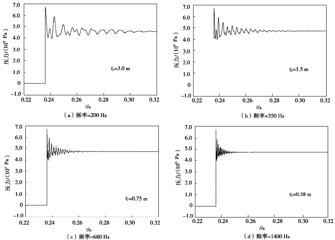
图 2 大于临界埋深时岩体内爆腔压力变化特点
