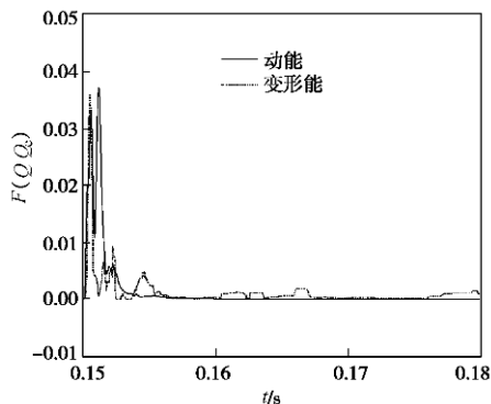
图9 动能和变形能变化图
