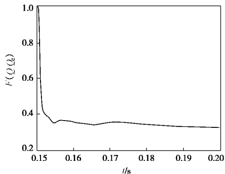
图8 爆破作用指数为1时内能变化图
