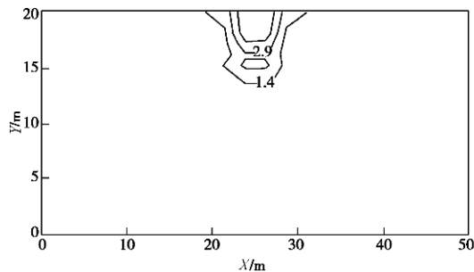
图7 标准的爆破漏斗模拟图
