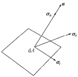
图 40 坡体潜在滑面受力示意图
