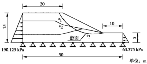
图 37 ACDAS 考题 EX1 (c) 计算模型
