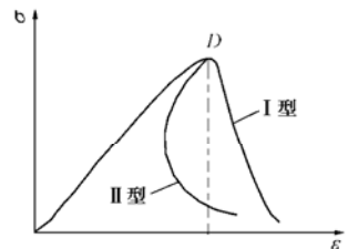
(b) 目前普遍采用的两类全过程曲线的基本模式
