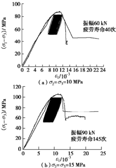
图 22 江西某地红砂岩三轴压缩的疲劳试验曲线与静态全过程曲线的关系图
