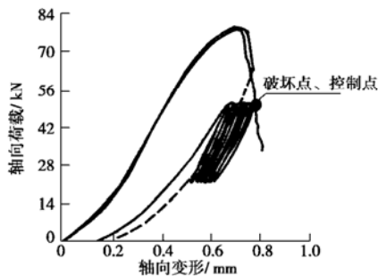
图 20 贵溪红砂岩峰值后区疲劳试验
