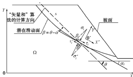
图 35 “矢量和”法安全系数求解示意图
