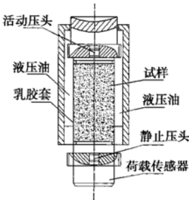
图 27 试样安装桶原理图
