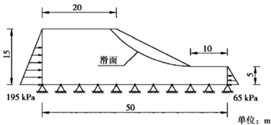
图 36 ACDAS 考题 EX1 (a) 计算模型
