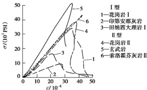
图2 6种岩石的单轴压缩试验曲线 [1]
