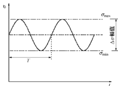
图11 周期加载波形
