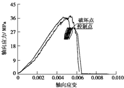
图 19 江西红砂岩#RS-6-1 试件峰后疲劳试件
