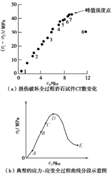
图 32 实测应力 - 应变全过程曲线与典型曲线对比
