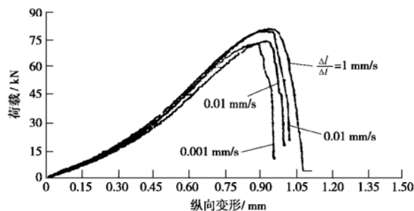
图 8 贵溪红砂岩在纵向变形率为 1 \sim 1 \times 10^{-3} \text{ mm/s} 时的全过程曲线簇
