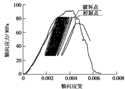
图 16 大冶大理岩 #M-2-1 试件疲劳试验曲线
