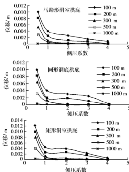
图7 拱顶位移与地应力的关系(不同埋深)
