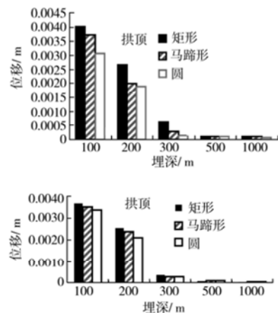
图 4 不同埋深下洞室位移随洞室断面变化情况 ( \lambda=2 )
