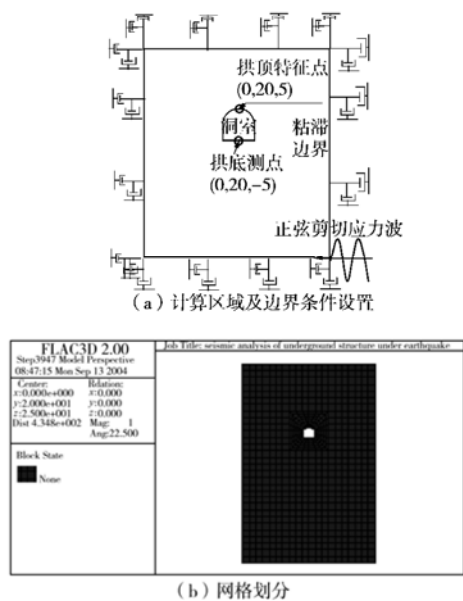
图1 计算模型
