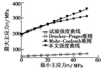
图1 岩石强度曲线比较
