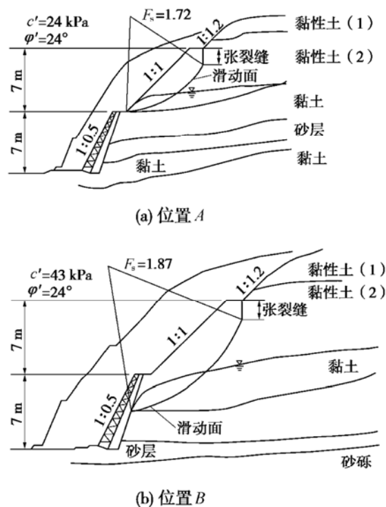
图2 人工切坡破坏实例
