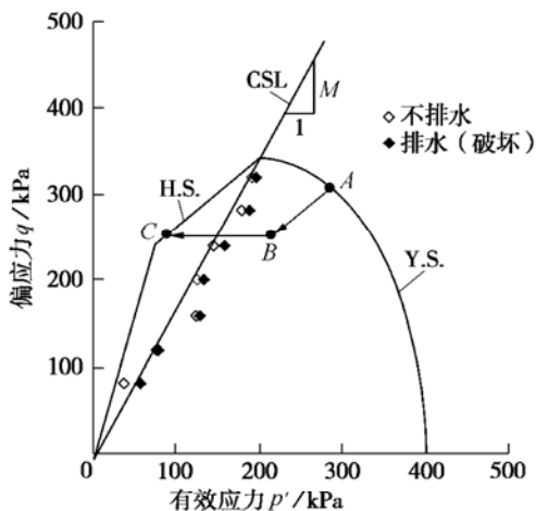
图 9 三轴试验结果
