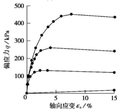
(b) 应力-应变曲线
