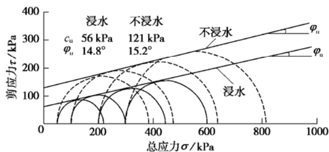
图6 UU试验结果
