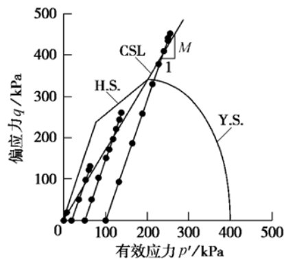
(a) 有效应力路径
