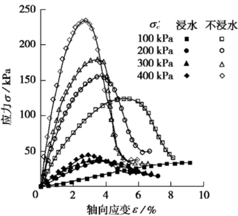
图 3 无侧限抗压强度试验结果 Fig. 3 Results of unconfined compression tests
