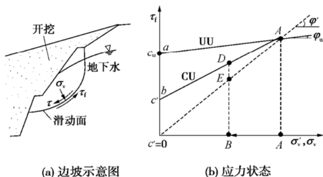
图1 切土边坡破坏与莫尔-库仑准则
