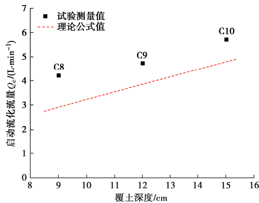
图 10 不同覆土深度的启动流化流量
