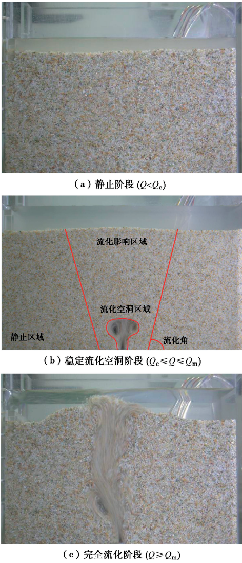
图 4 不同管道渗漏流量下的砂土流化现象
