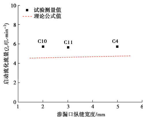
图 11 不同渗漏口尺寸的启动流化流量
