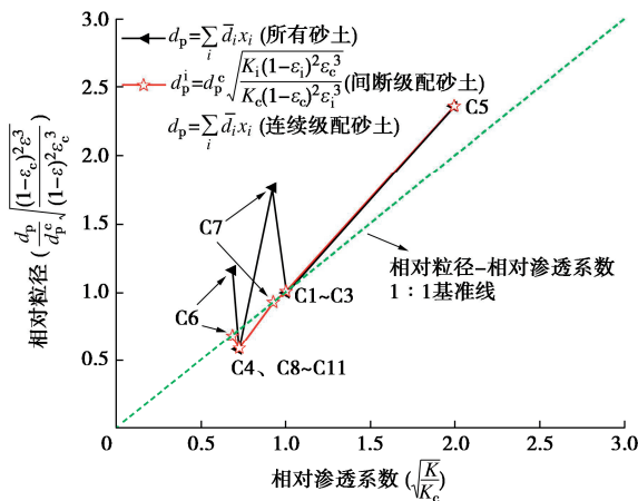
图 5 平均粒径计算值对比
