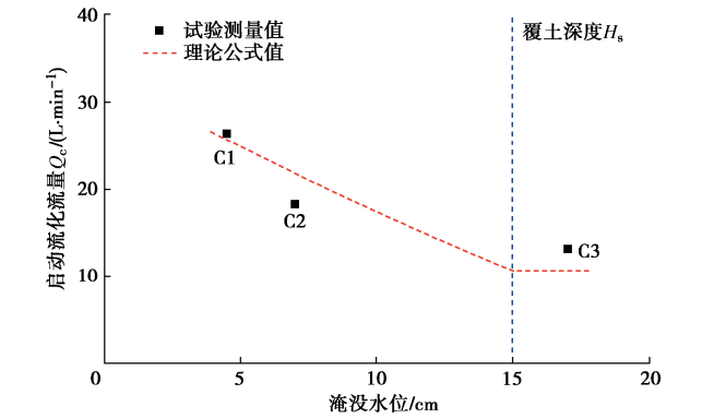
图 8 不同淹没水位的启动流化流量
