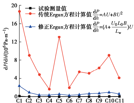
图 6 压力梯度试验值与公式计算值对比
