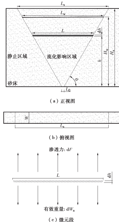
图 1 供水管道渗漏上部砂土流化区域示意图
