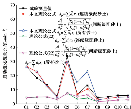
图 7 启动流化流量理论计算值与试验测量值对比
