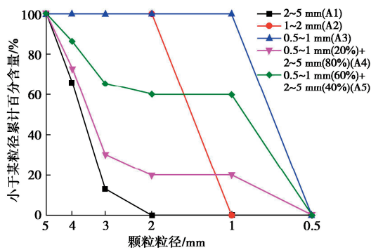
图 3 颗粒级配曲线 Fig. 3 Particle size distribution curves
