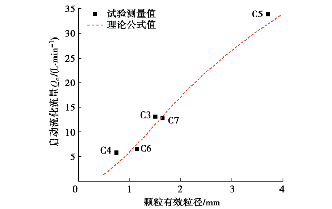
图 9 不同颗粒有效粒径的启动流化流量
