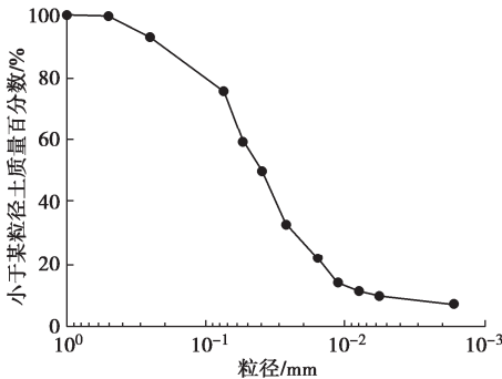
图 1 青海粉质黏土级配曲线
