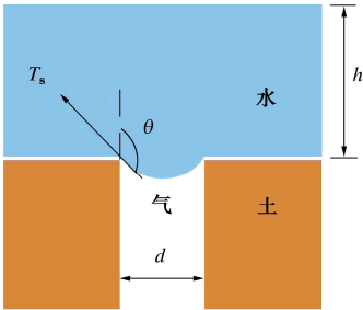
(b) 疏水材料中的毛细作用
