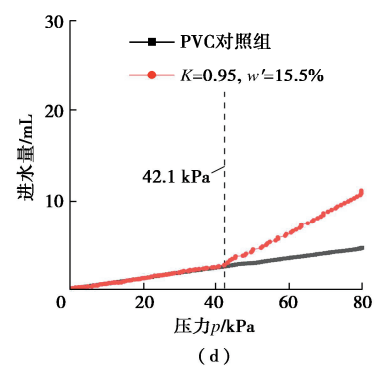
图 7 土样进水量-压力关系曲线 (以压实度 0.95 为例)
