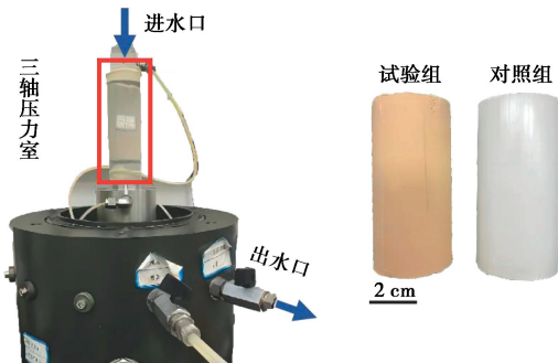
图 5 击穿压力试验装置及试样
