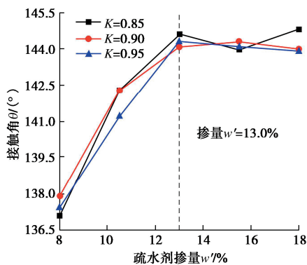
图 6 疏水剂掺量-接触角关系
