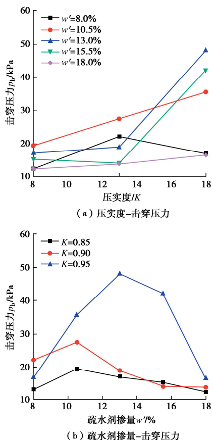
图 8 压实度和疏水剂掺量对疏水土击穿压力的影响
