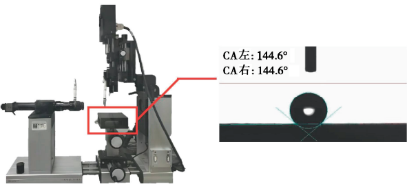
图 3 接触角测量示意图
