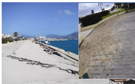
图 2 2014 年希腊地震 Cephalonia 岛砾石喷出地表,砾性土液化导致堤岸侧移 [10]
