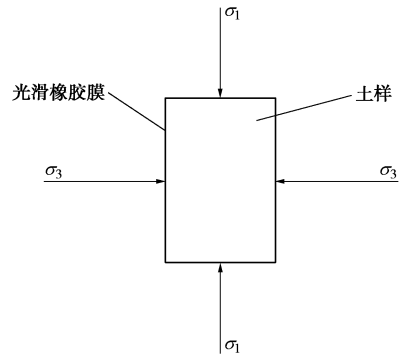
图1 土的常规三轴压缩试验示意图
