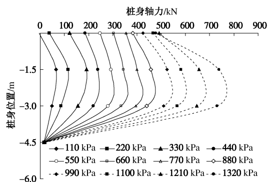
图 5 复合地基中 PHC 桩桩身轴力典型分布
