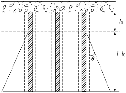
图 7 复合地基应力扩散模型
