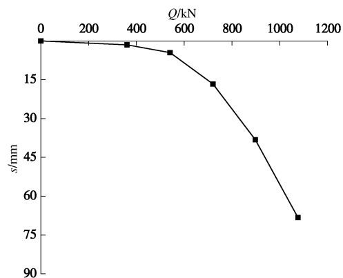
图 2 PHC 桩单桩静载荷试验 Q-s 曲线
