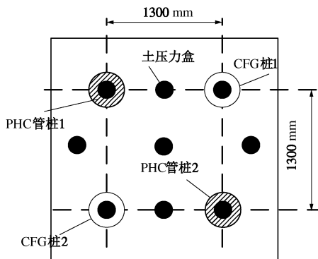
(d) 土压力盒测点布置
