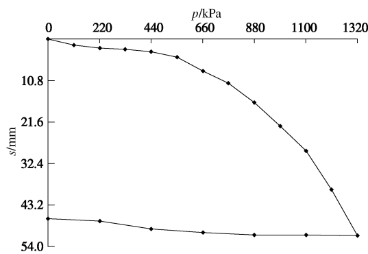
(b) 第二组 4 桩组合式长短桩复合地基静载荷试验 p-s 曲线
