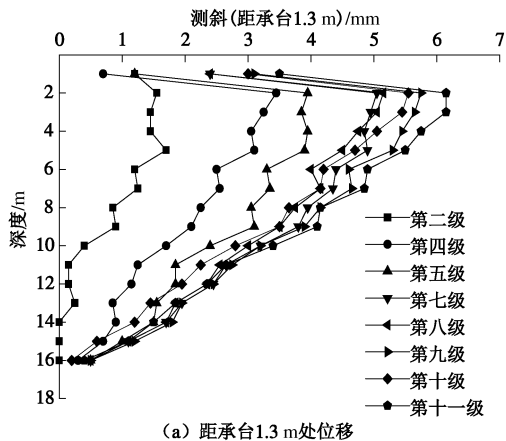
(a) 距承台 1.3 m 处位移
