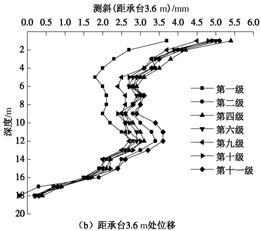
图 6 深层土体侧向位移曲线
