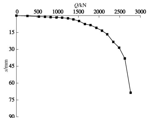
图 3 CFG 桩单桩静载荷试验 Q-s 曲线
