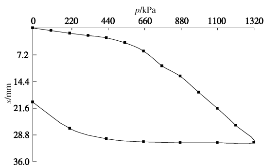
(a) 第一组 4 桩组合式长短桩复合地基静载荷试验 p-s 曲线
